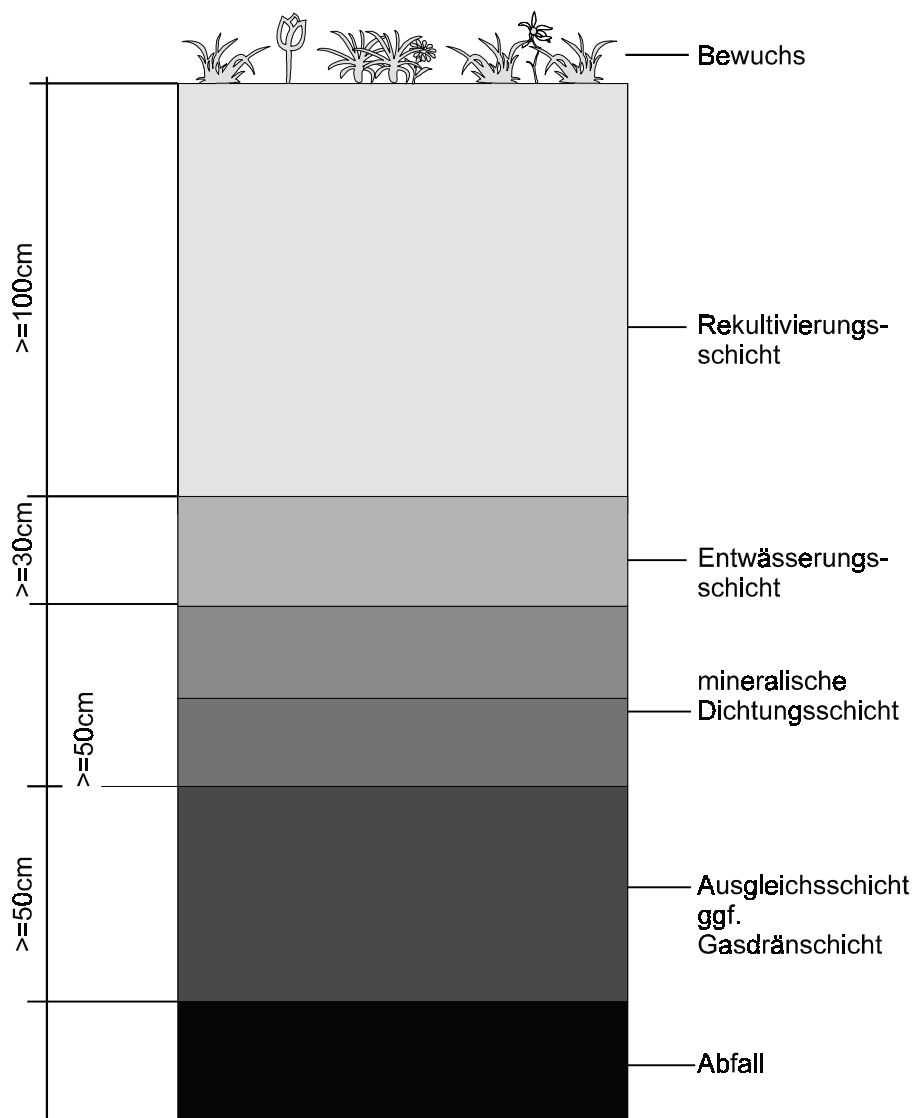
Bild 2: Deponieoberflächenabdichtungssysteme
