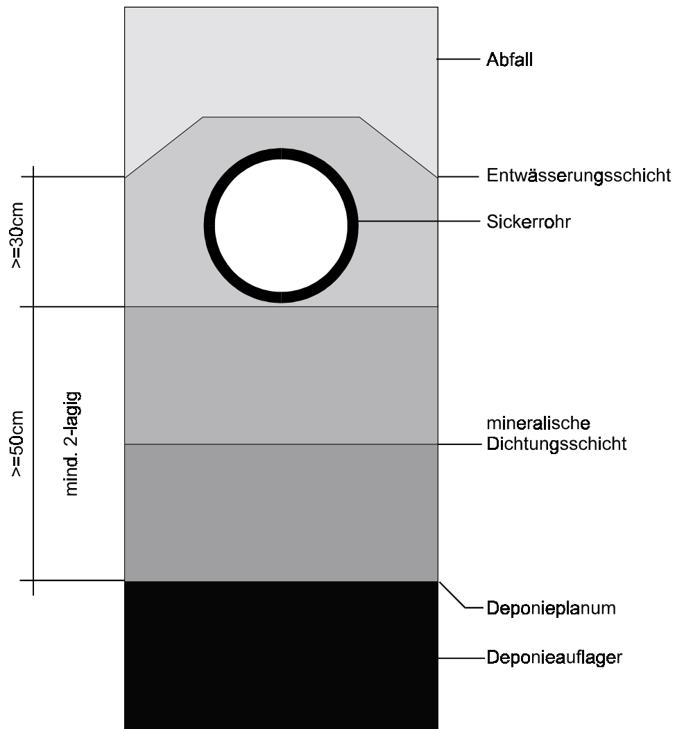
Bild 1: Deponiebasisabdichtungssysteme
